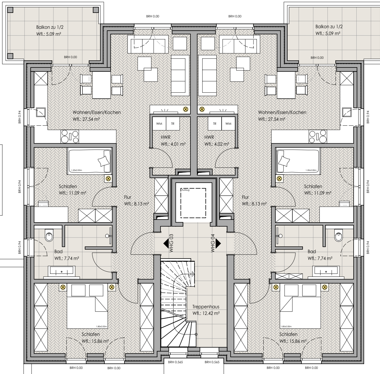
Grundriss 1. Obergeschoss Haus Nr. 2a
