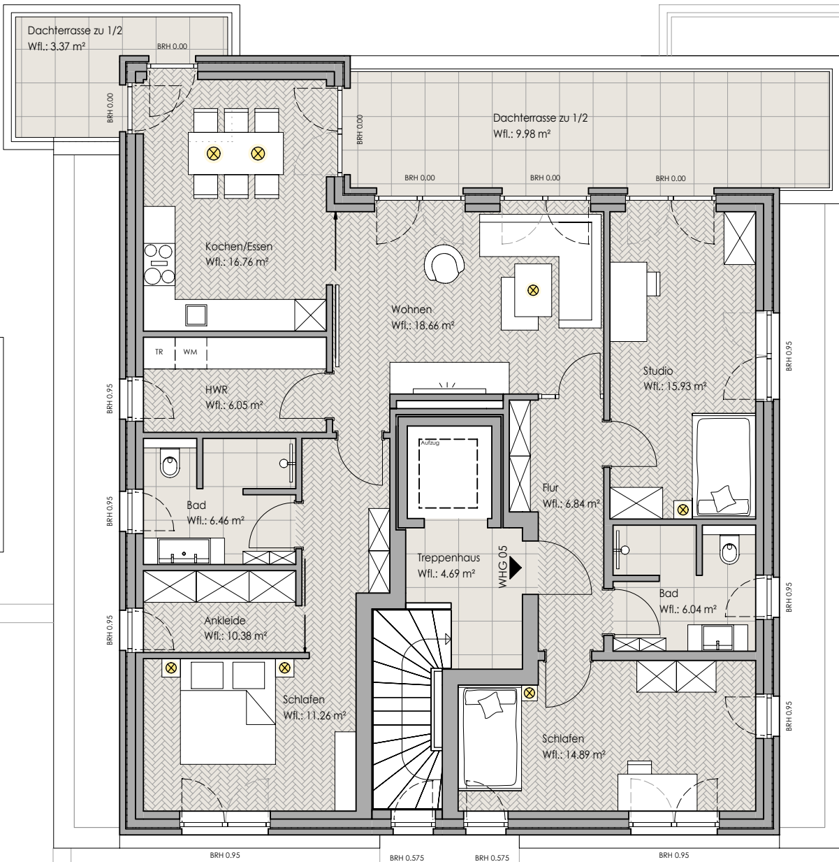
Grundriss 2. Obergeschoss Haus Nr. 2a
