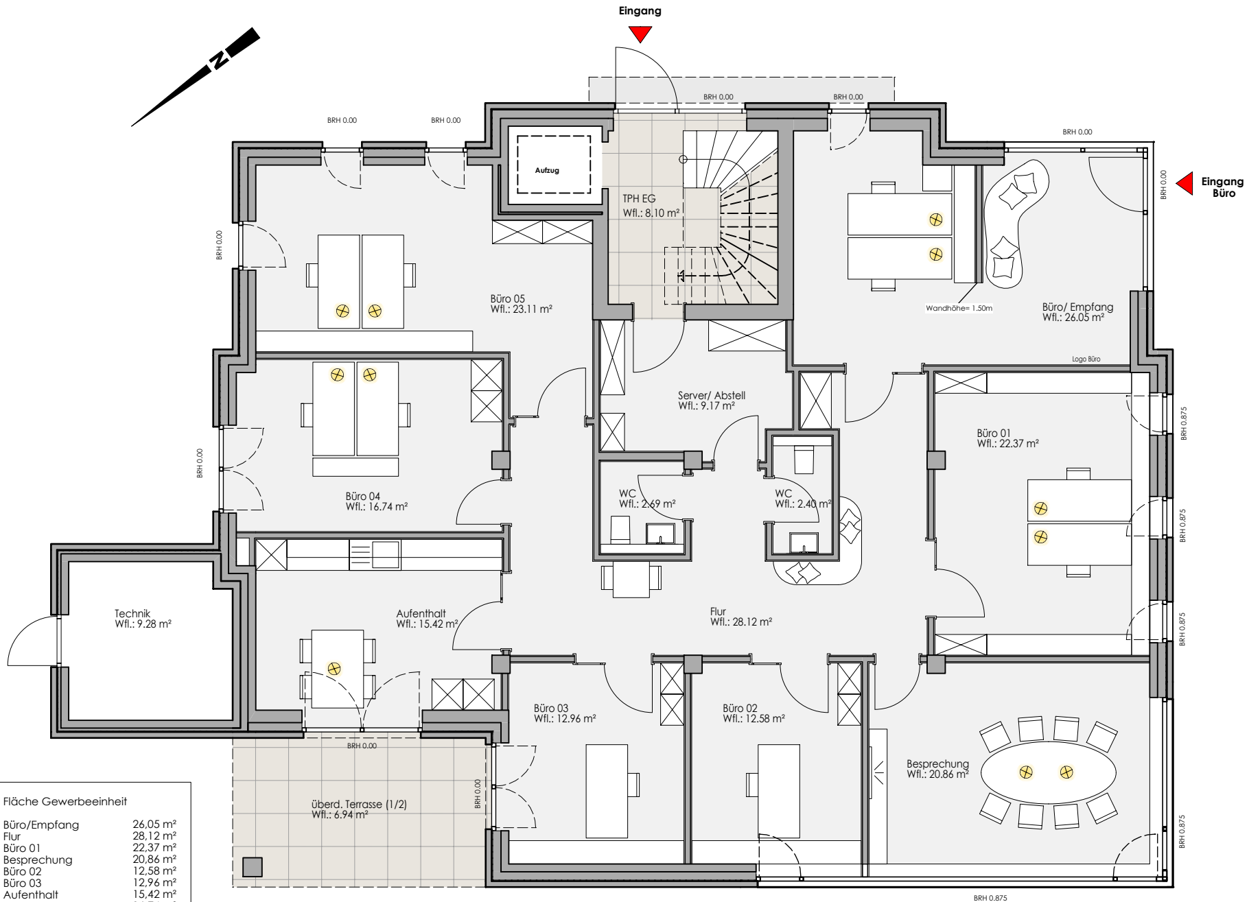
Beispielgrundriss Erdgeschoss Haus 01
