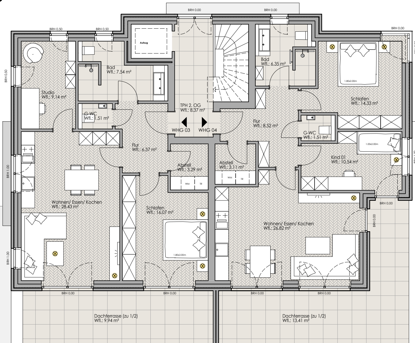
Grundriss 2. Obergeschoss Haus 02
