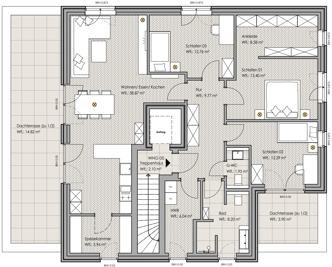
Grundriss 2. Obergeschoss Haus 04
